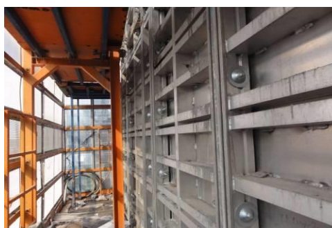
图 3.4-2 爬模模板及架体
